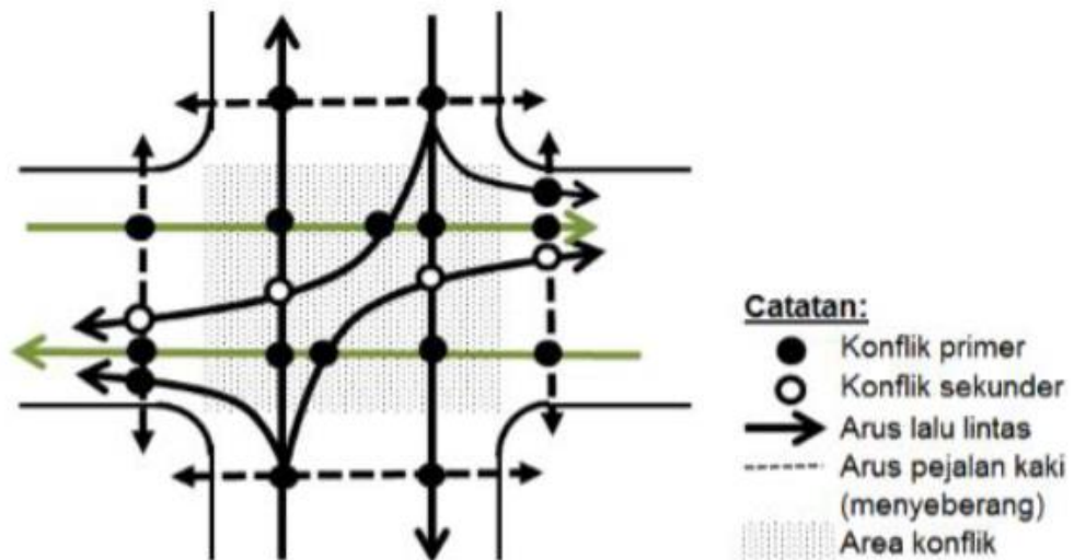
Gambar 6.1 Konflik Primer dan Sekunder
