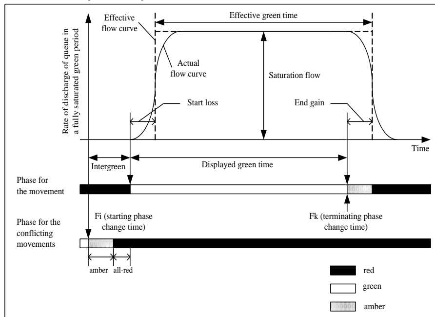
Gambar 6.3 Model Dasar Arus Jenuh
