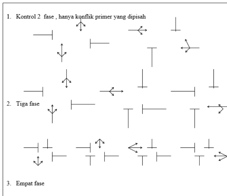
Gambar 6.2. Fase Dasar untuk Pemisahan Konflik Primer
