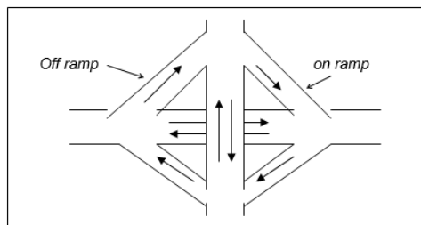
Gambar 5.2 Persimpangan Tidak Sebidang
