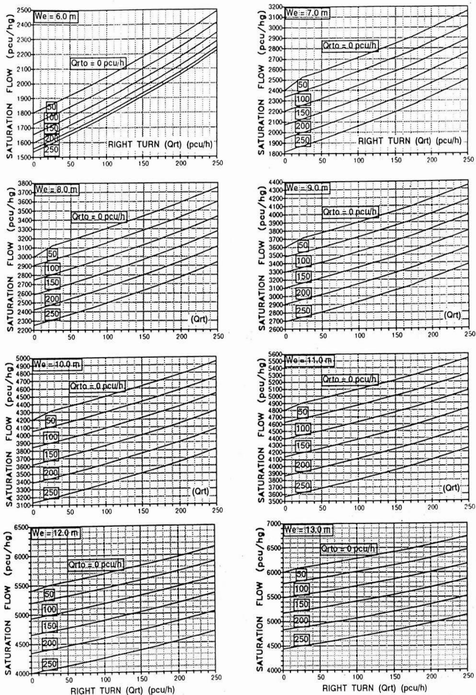
Gambar Arus Jenuh Dasar Pendekat Tipe O Dengan lajur Belok Kanan Terpisah
