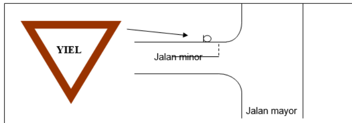
Gambar 5.11. Persimpangan dengan Yield Signs/Give Way Sign
