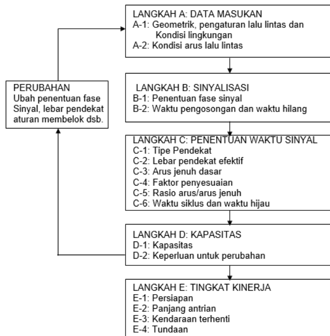
Gambar 6.5. Bagan Alir untuk Analisis APILL
