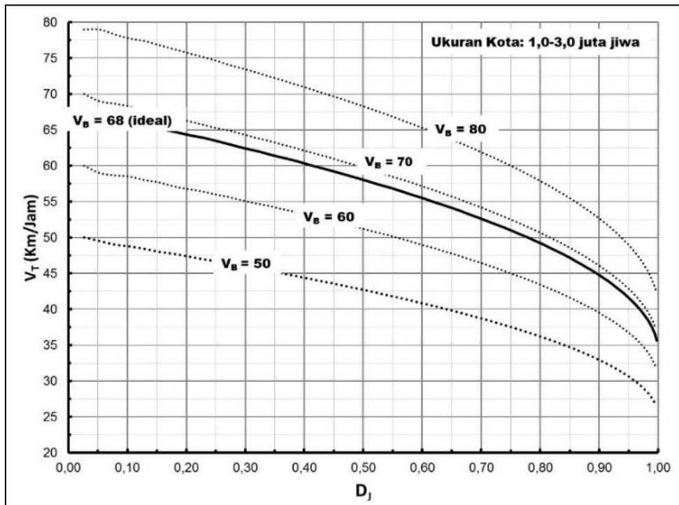
Gambar 4.2b Kecepatan Sebagai Fungsi Q/C Jalan 4/2T, 6/2T
