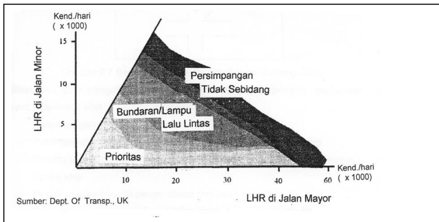
Gambar 5.4. Penentuan Penanganan Persimpangan
