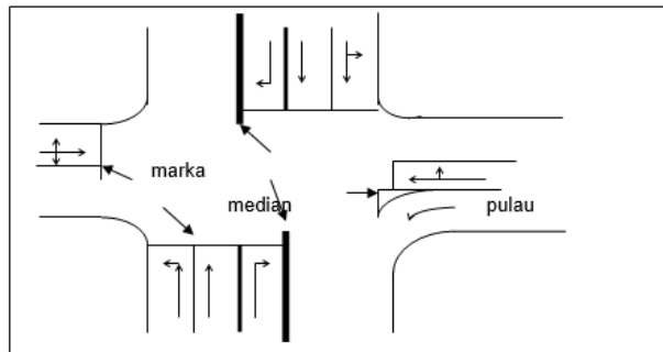
Gambar 5.13 Persimpangan dengan Pengaturan Kanalisasi
