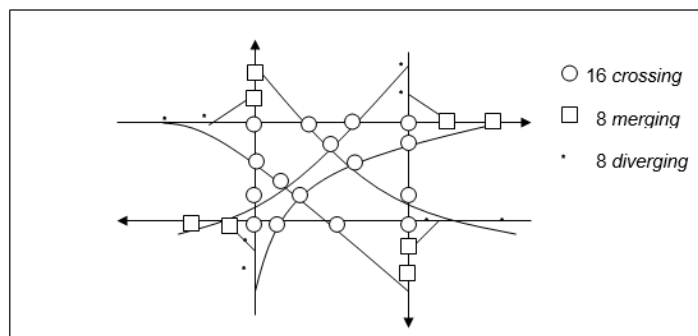
Gambar 5.9 Titik-titik konflik pada persimpangan 4 kaki.
