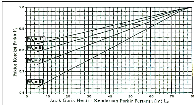
Gambar Faktor Penyesuaian Untuk Pengaruh Parkir dan Jalur Belok Kiri yang Pendek ( F_p )
