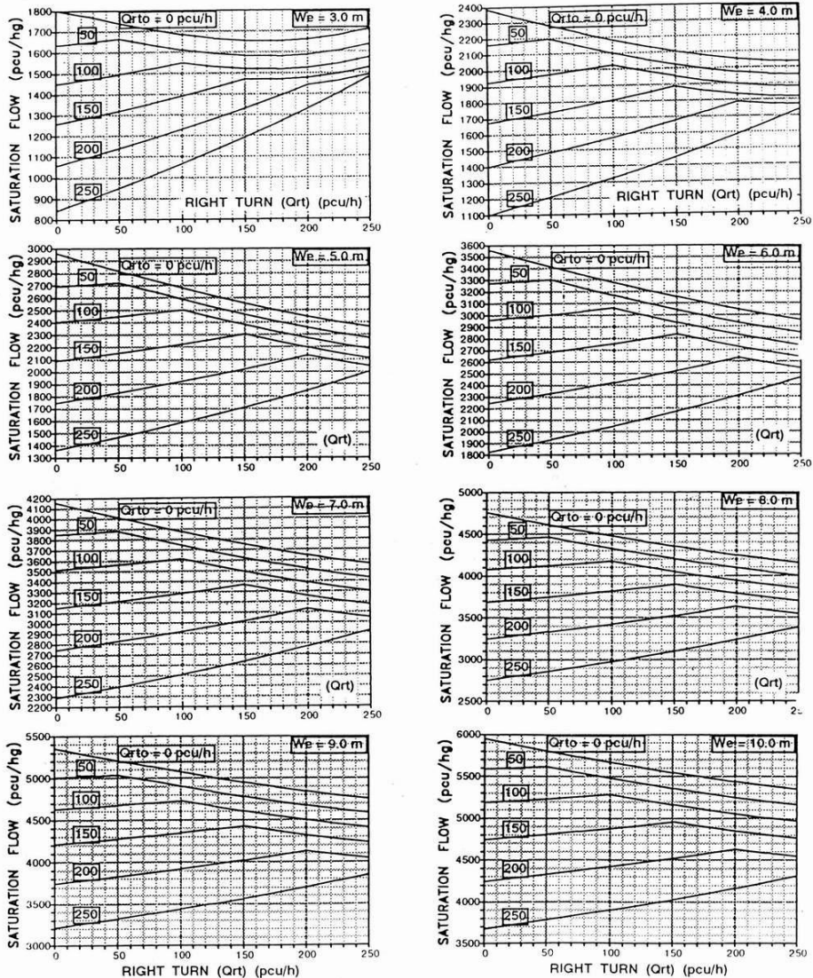
Gambar Arus Jenuh Dasar Pendekat Tipe O Tanpa lajur Belok Kanan Terpisah
