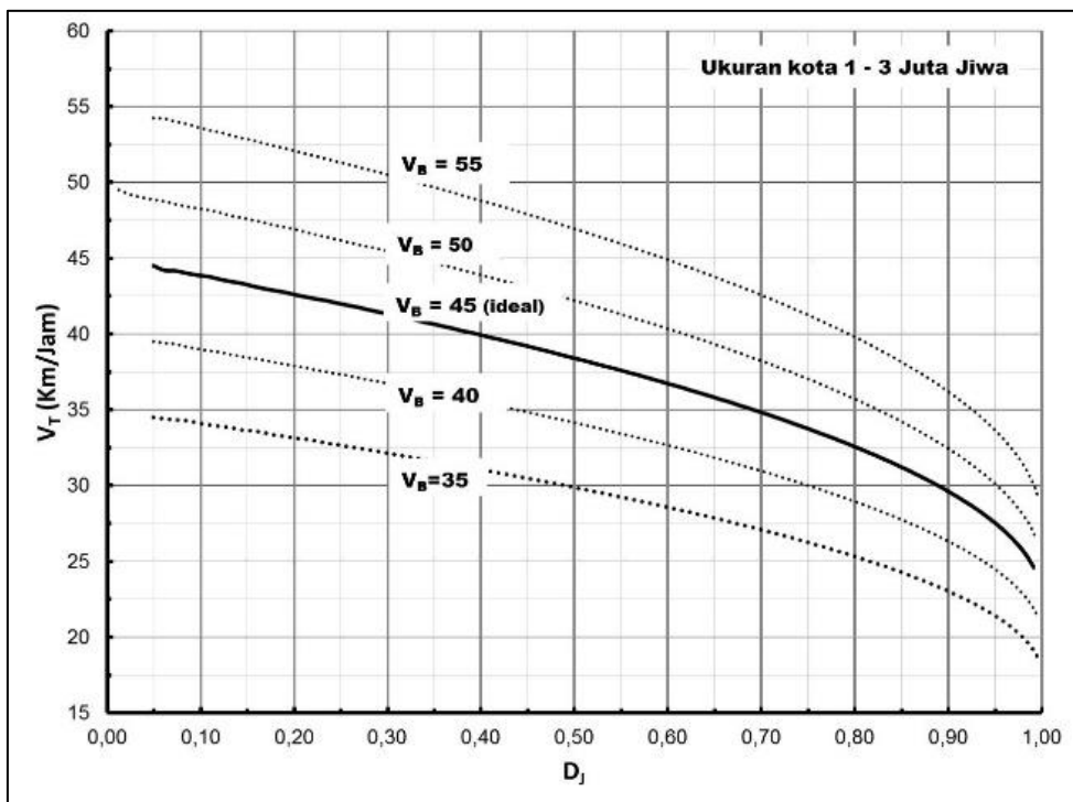
Gambar 4.2a Kecepatan Sebagai Fungsi Q/C Jalan 2/2 TT
