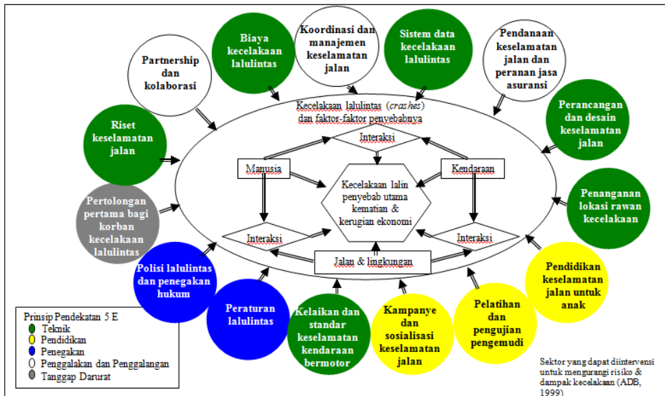
Gambar 8.1. Sektor Keselamatan Lalulintas (Dephub, 2008)
