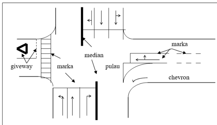
Gambar 7.1 Beberapa jenis Marka Jalan
