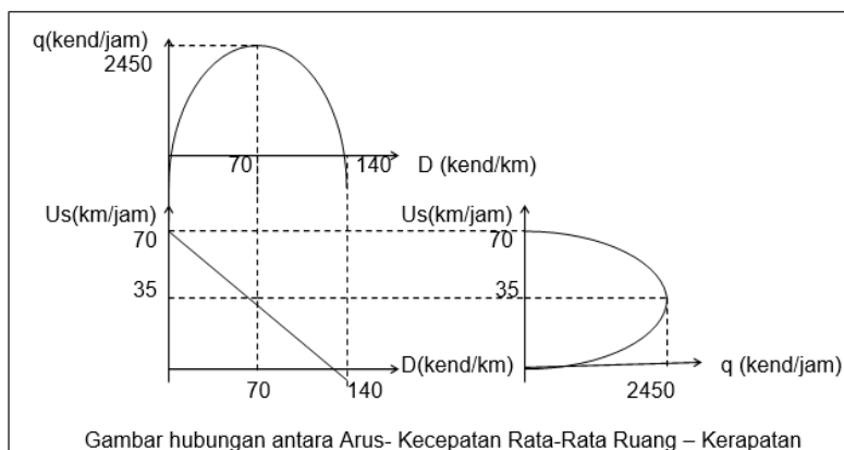
Gambar hubungan antara Arus- Kecepatan Rata-Rata Ruang – Kerapatan
