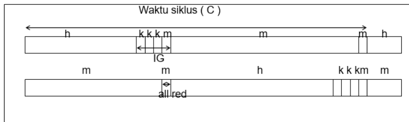
Gambar 6.4 Diagram waktu
