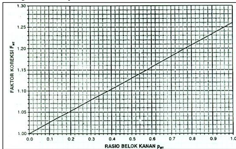
Gambar Faktor Penyesuaian Untuk Belok Kanan ( F_{RT} )
